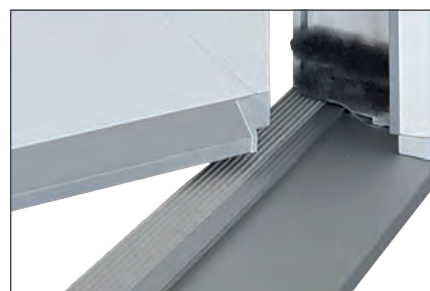
Wetterschenkel seitlich verschlossen Bodenschwelle thermisch getrennt
