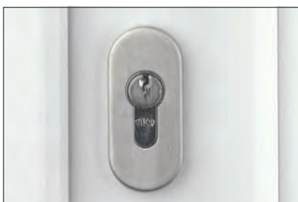
Ovale Rosette aus Edelstahl auf der Außenseite, inkl. Profilzylinder mit Not- und Gefahrenfunktion (Aufschließen trotz innen steckenden Schlüssels)
