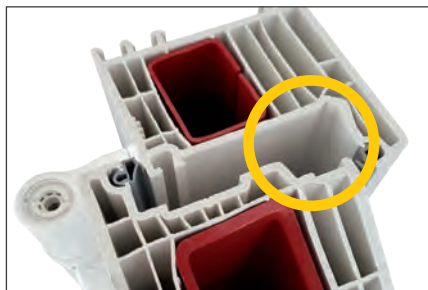
Wandungsstärke bis 3,5 mm für optimale Stabilität
